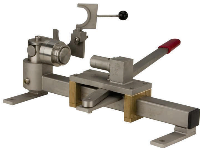
Drum Valve Montagewerkzeug für Ventile 741-093
