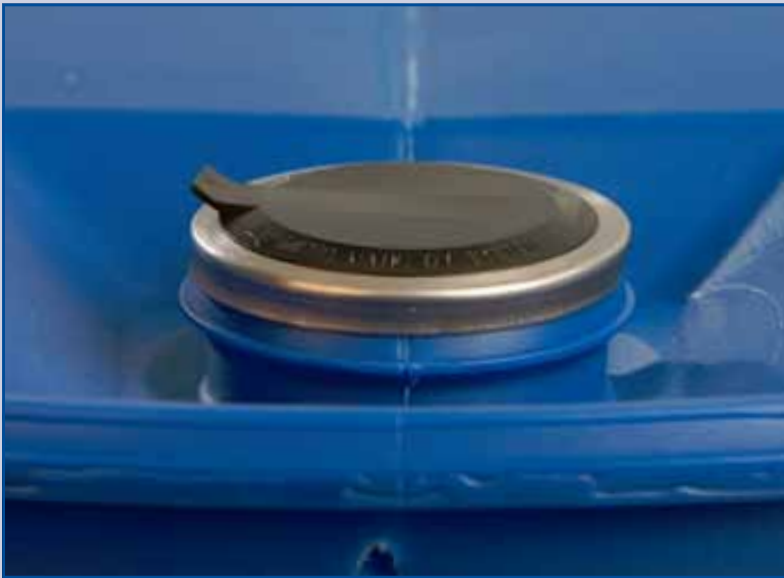
56x4 mit Clinchring und Originalitätsverschluß.
